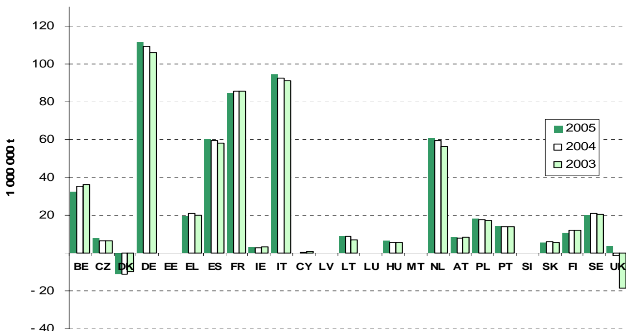
Abbildung 2: Nettoeinfuhren von Rohöl
