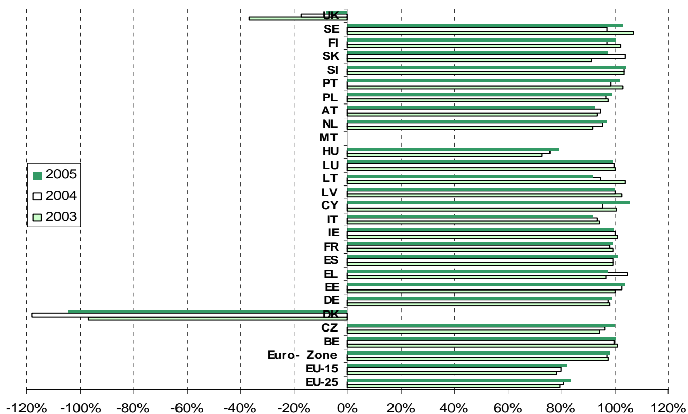
Abbildung 3: Energieabhängigkeit – Erdöl (Rohöl und Mineralölerzeugnisse)
