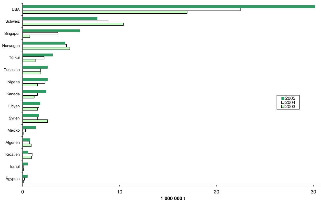
Abbildung 5: Ausfuhren von Mineralölzeugnissen (Extra-EU) insgesamt
