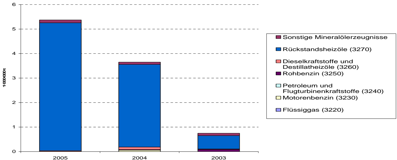
Abbildung 9: Ausfuhren von Mineralölzeugnissen nach Singapur insgesamt
