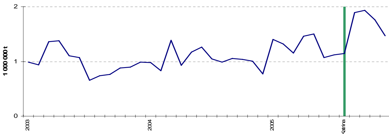
Abbildung 6: Ausfuhren von Motorenbenzin in die USA (Januar 2003 bis Dezember 2005)
