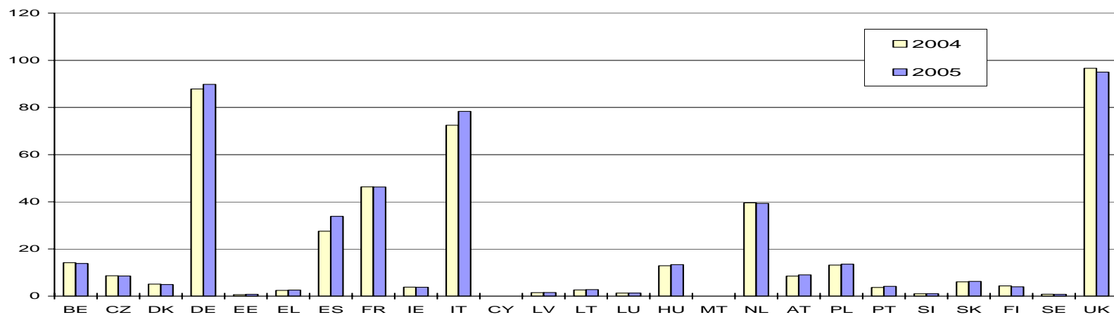
Abbildung 2: Bruttoinlandsverbrauch in Mio. tRÖE (Ho)
