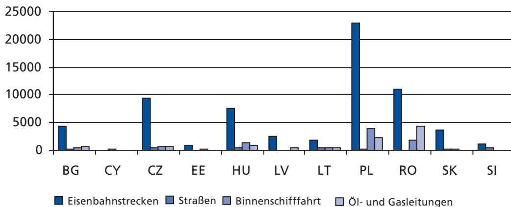
Abbildung III. 18.1 - Eisenbahnstrecken, Straßen, Binnenschifffahrt und Öl- und Gasleitungen in den Beitrittsländern, in Kilometer, 1999
