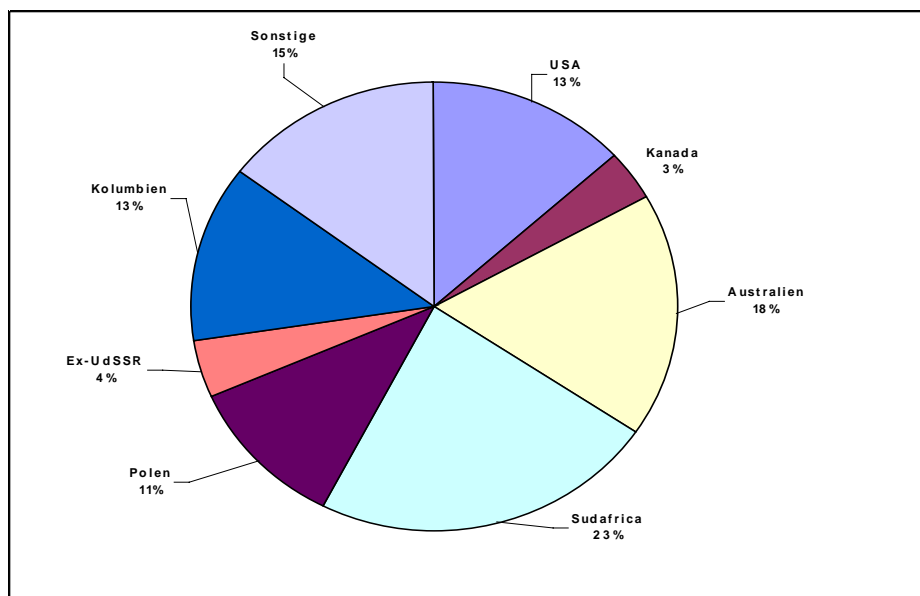
Abbildung 1: Steinkohlenimporte EU nach Herkunft, 1999
